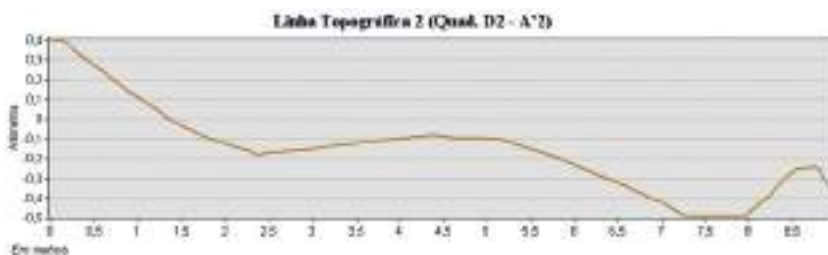
Figura 14 – Linha topográfica superficial 2.
